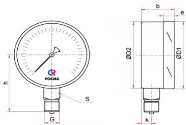
Радиальное присоединение
